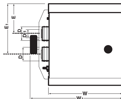
نمای جانبی
